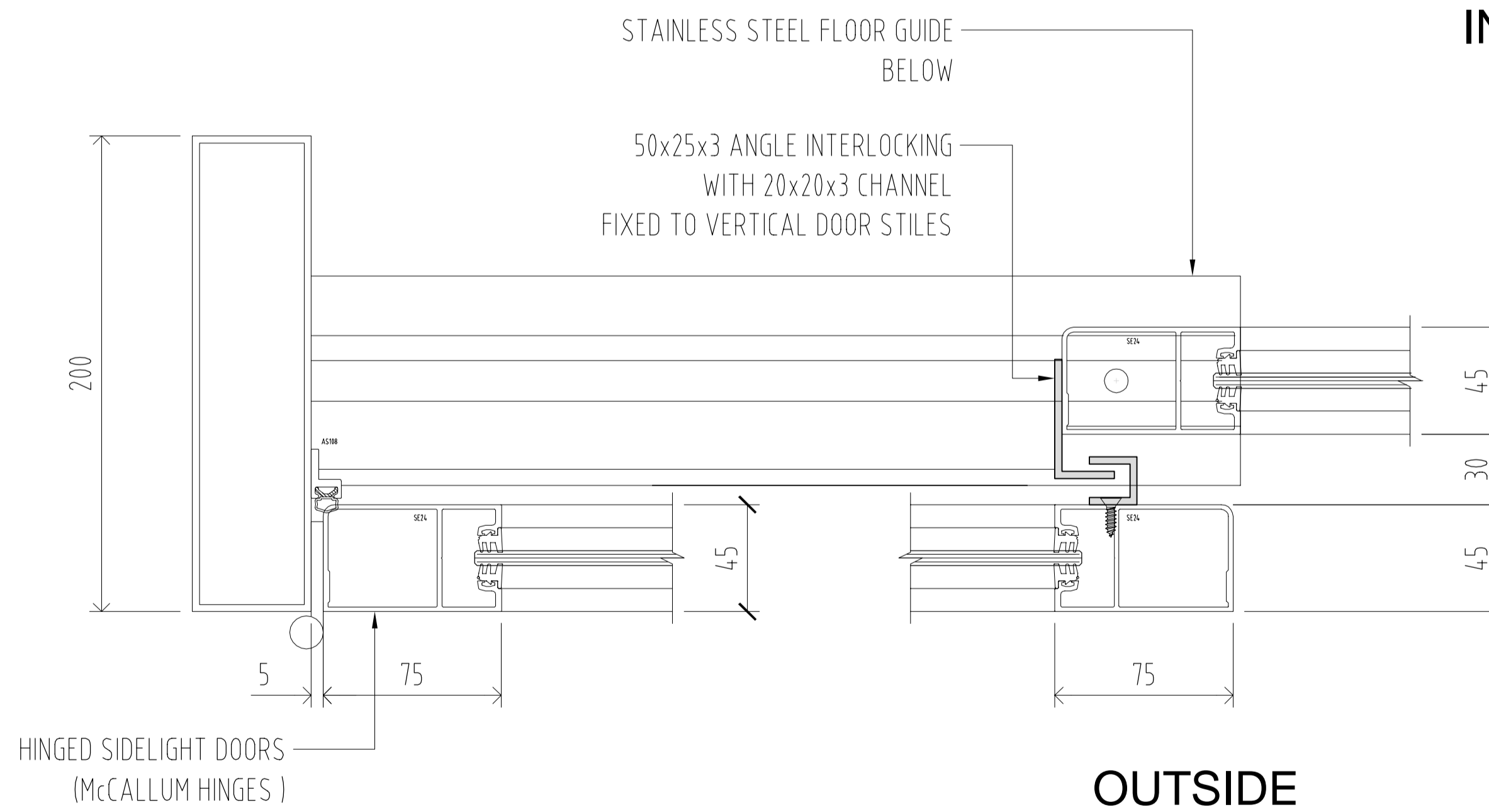
B 009 PLAN DETAIL SCALE: 1:2
