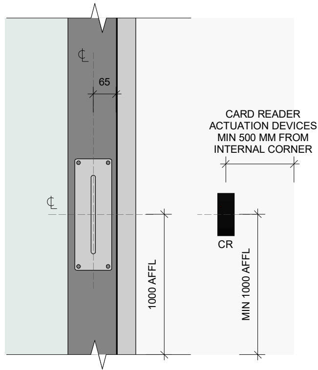
SGL0012-A PULL SIDE
